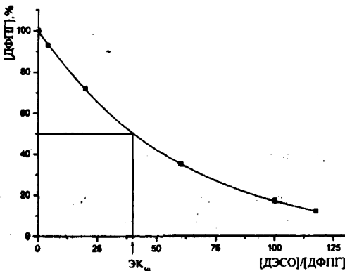
Рис. 3. Зависимость нереагировавшей части ДФПГ (в %) от отношения концентраций ДЭСО и ДФПГ.
