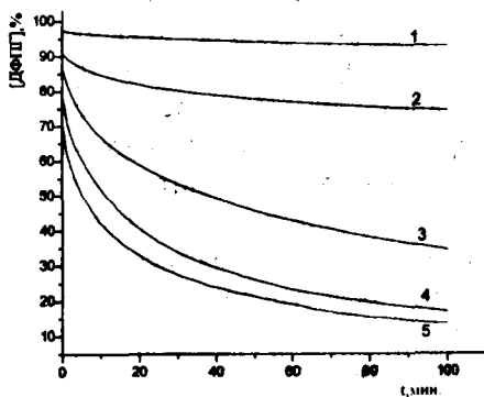
Рис. 2. Кинетические кривые взаимодействия ДФПГ с ДЭСО (в %) в метаноле, где [ДФПГ] = 0,525 \cdot 10^{-4} M , [ДАСО]/[ДФПГ] : 1 – 4 \cdot 10^3 , 2 – 20 \cdot 10^3 , 3 – 60 \cdot 10^3 , 4 – 100 \cdot 10^3 , 5 – 117,5 \cdot 10^3 M .
